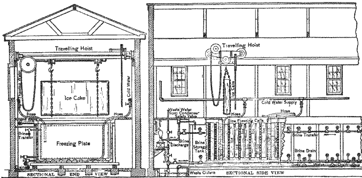
FIG. 236.—Plate Ice-tank.
